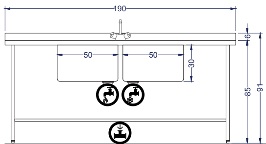
Vista Elevación
