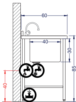
Vista Izquierda
