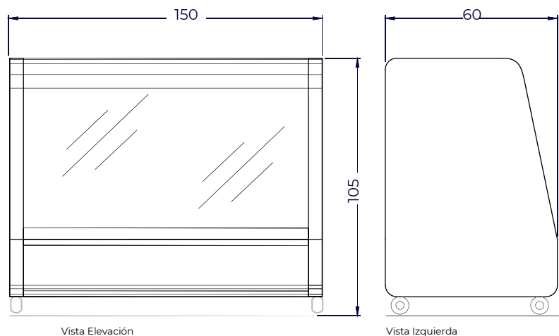
Vista Elevación
