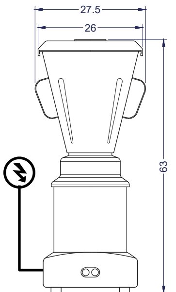
Vista Elevación
