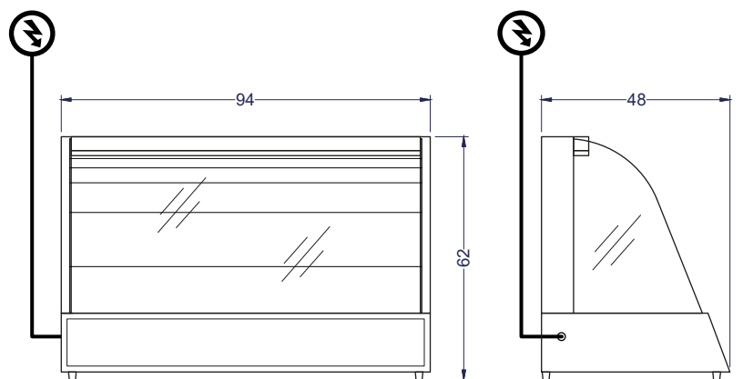
Vista Elevación
