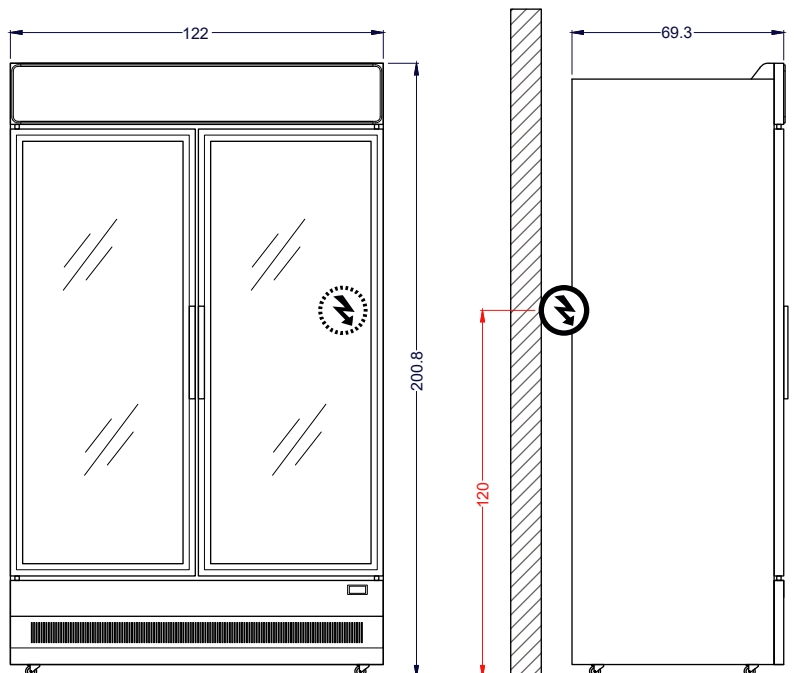
Vista Elevación
