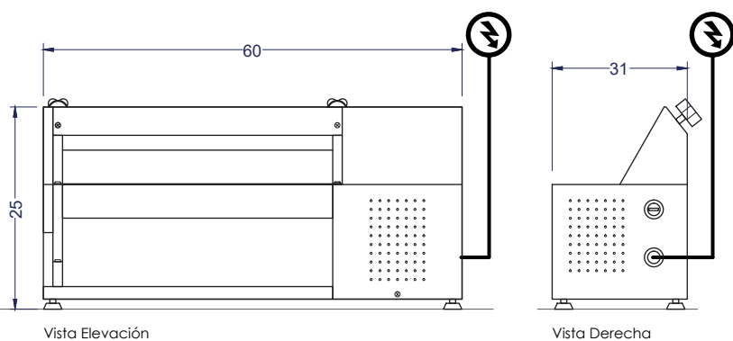
Vista Elevación
