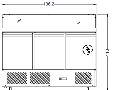
Vista Elevación
