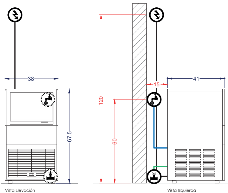
Vista Elevación
