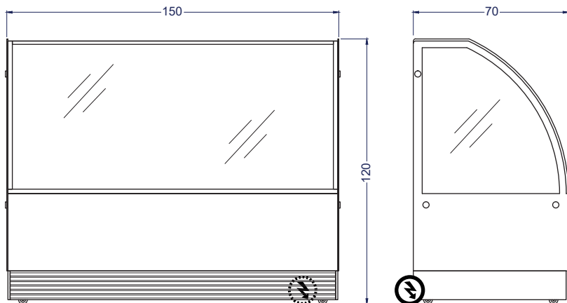
Vista Elevación
