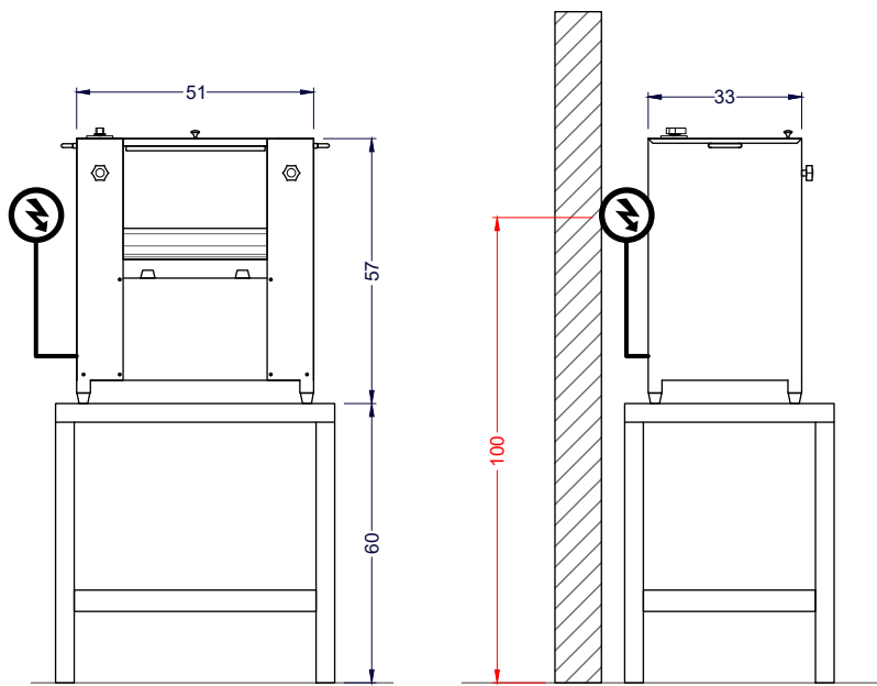
Vista Elevación
