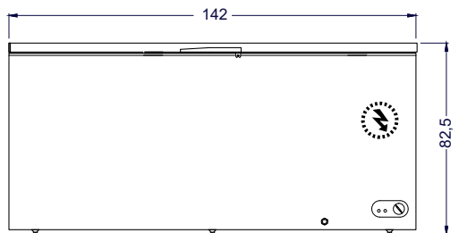
Vista Elevación
