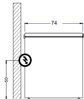
Vista Izquierda
