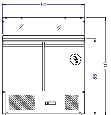
Vista Elevación
