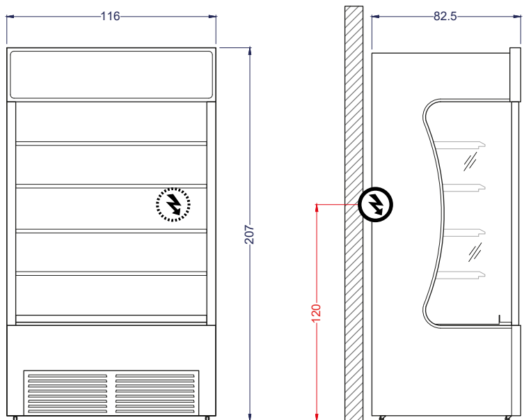
Vista Elevación
