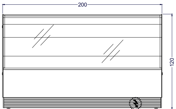
Vista Elevación
