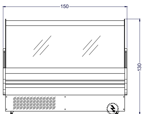
Vista Elevación
