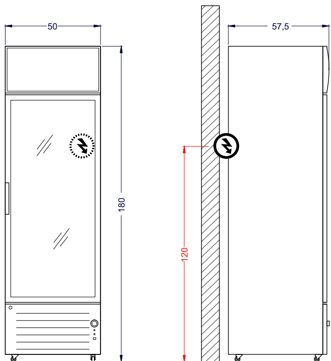
Vista Elevación
