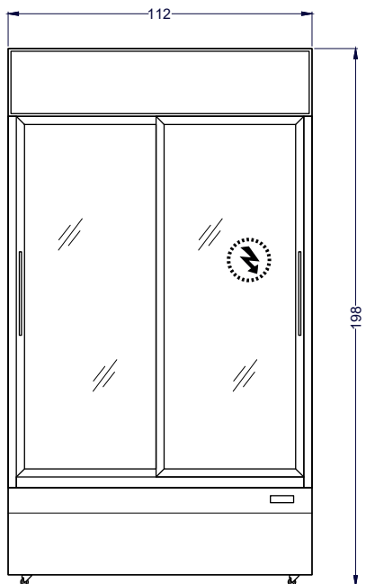
Vista Elevación
