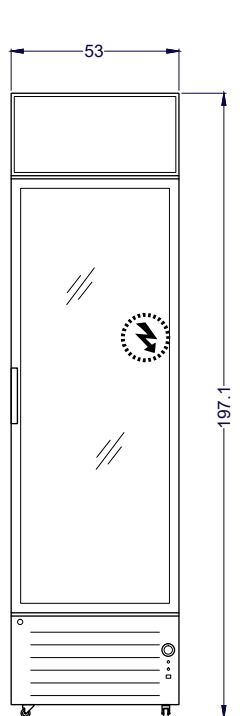
Vista Elevación
