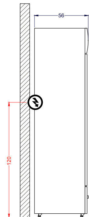
Vista Izquierda
