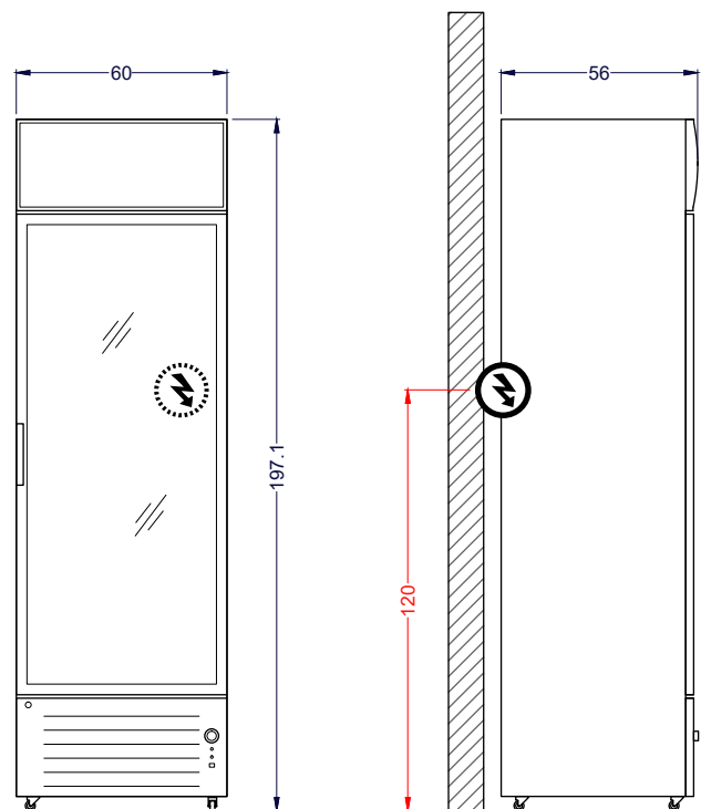
Vista Elevación
