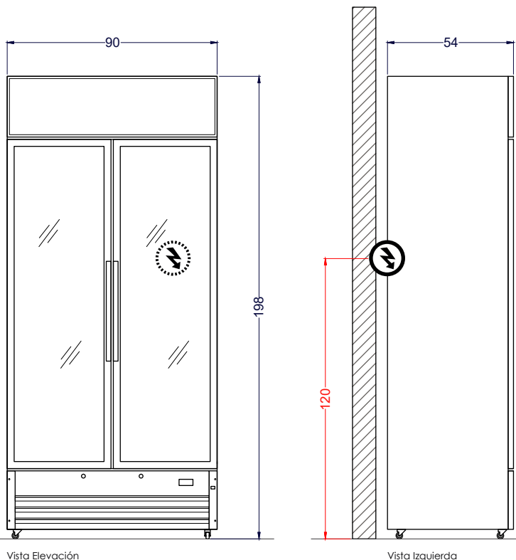
Vista Elevación
