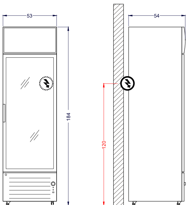
Vista Elevación
