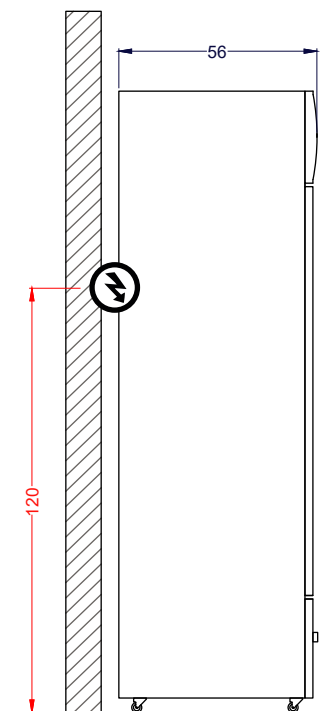
Vista Izquierda
