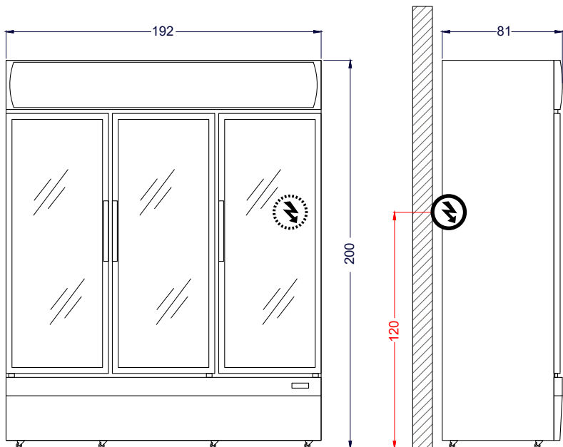
Vista Elevación
