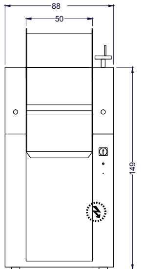
Vista Elevación
