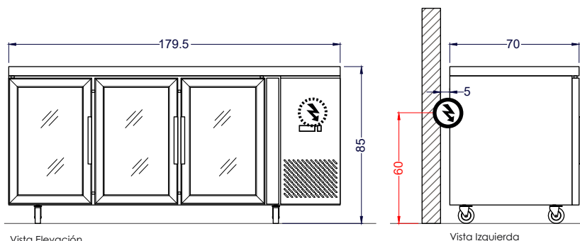
Vista Elevación
