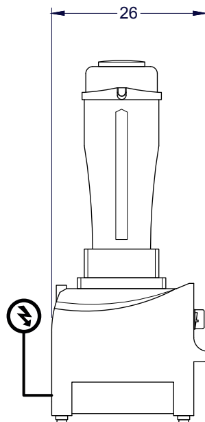
Vista Izquierda
