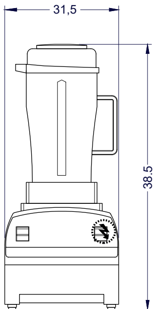
Vista Elevación
