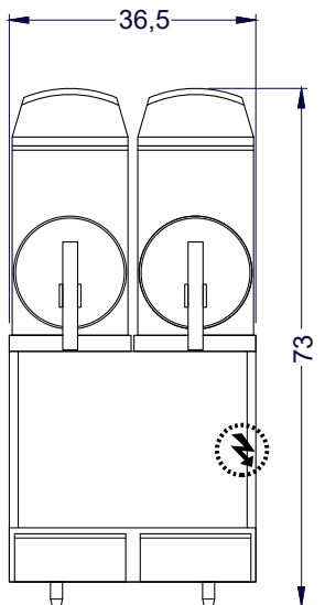
Vista Elevación
