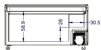
Vista Elevación
