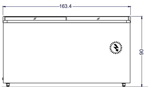
Vista Elevación
