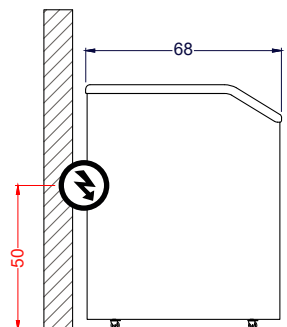
Vista Izquierda
