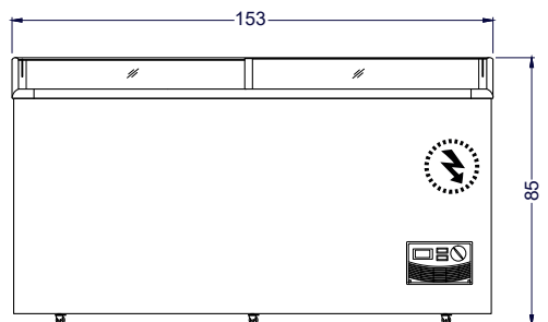
Vista Elevación
