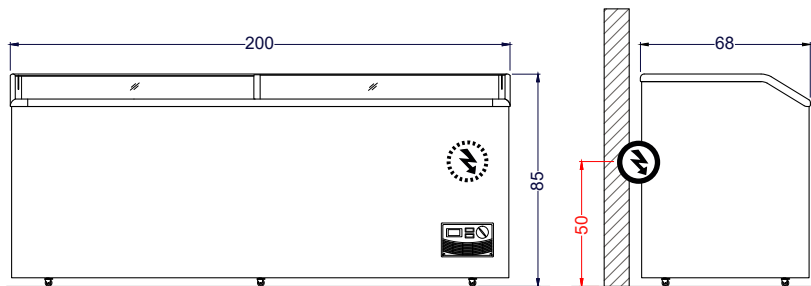
Vista Elevación
