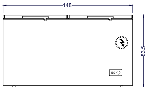
Vista Elevación
