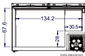
Vista Elevación
