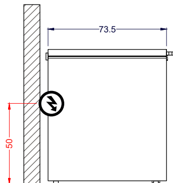
Vista Izquierda
