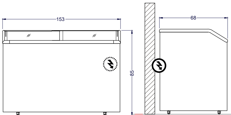
Vista Elevación
