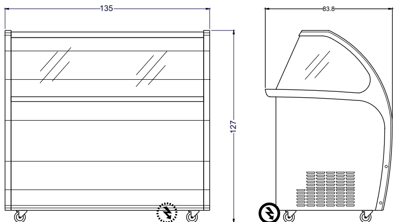
Vista Elevación
