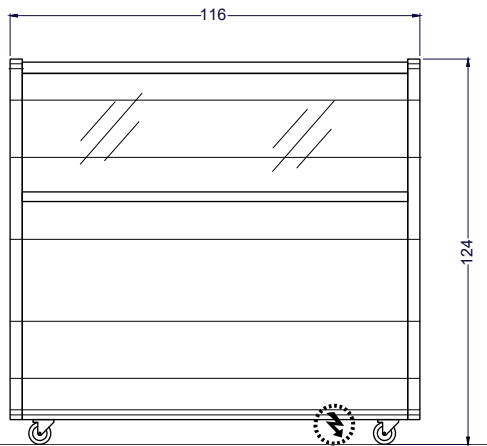
Vista Elevación
