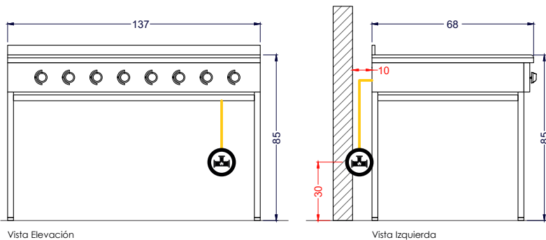
Vista Elevación
