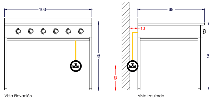
Vista Elevación
