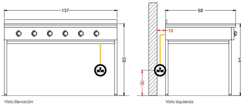
Vista Elevación
