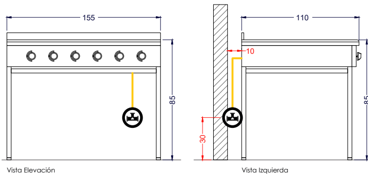
Vista Elevación
