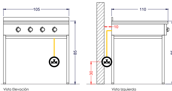
Vista Elevación
